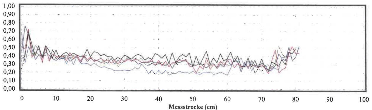
Gleitreibungskoeffizient [μ]
